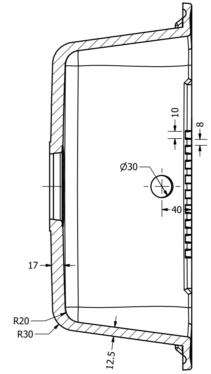
PRZEKRÓJ C-C SKALA 1 / 3
